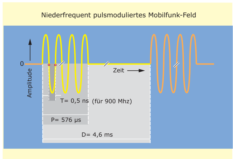
Bild 7: Typische zeitliche Abläufe der niederfrequent gepulsten Mikrowellen des Mobilfunks im D-Netz
